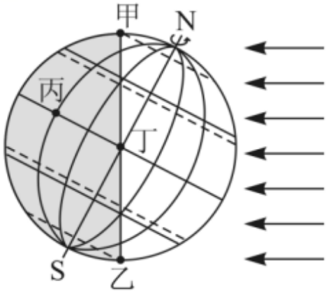
西半球某日的光照图
