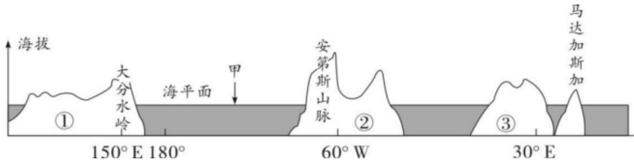
沿 23° 26'S 地形剖面示意图
